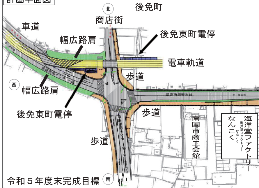
後免東町交差点の改良工事、完成予定図（県ホームページより作成）
